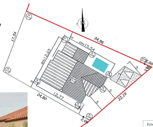
Un plan de masse*
